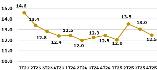
ROE 12M (%)
